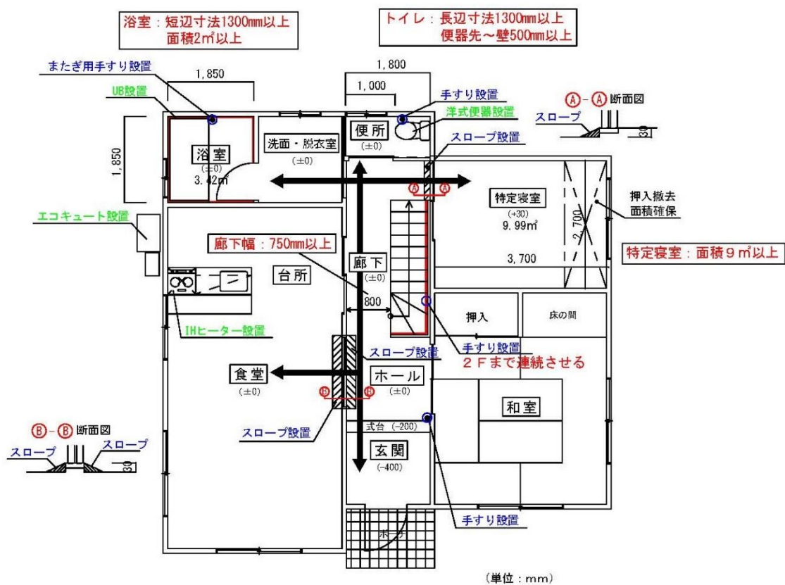
改修後 1階平面図
