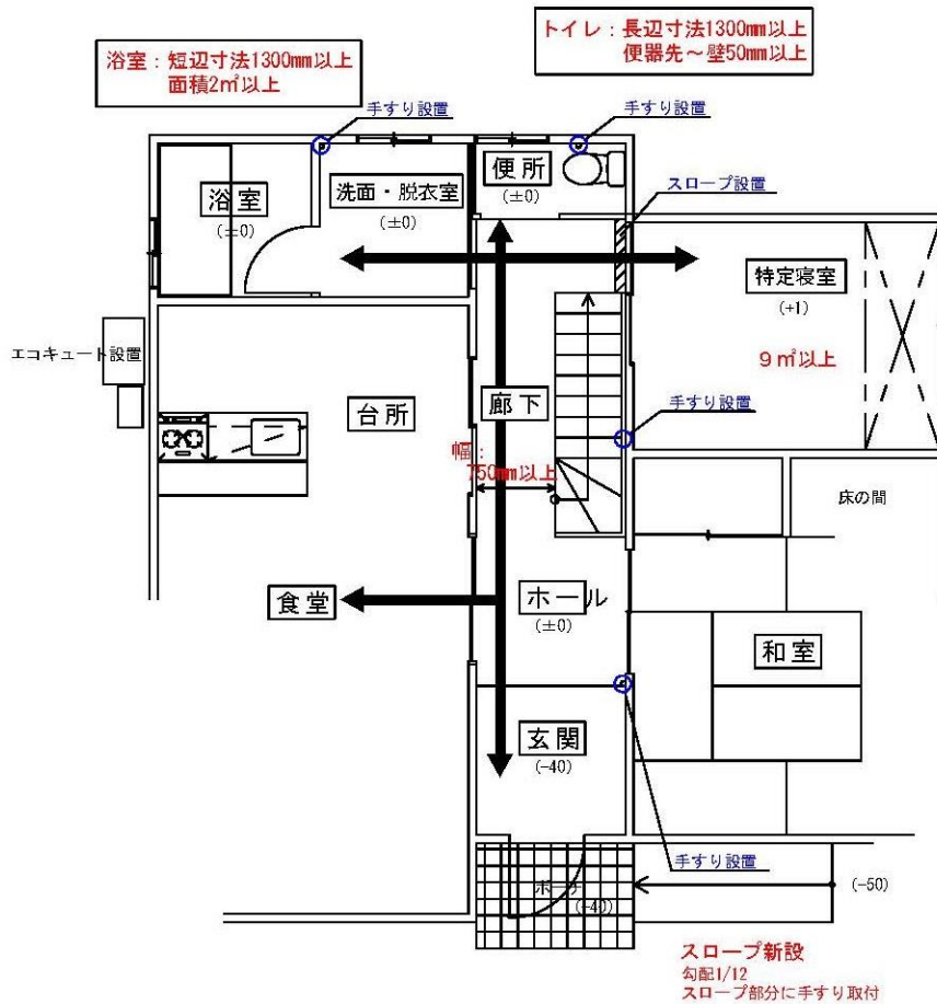
1階平面図 1/100
